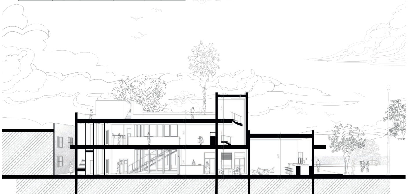
Coupe longitudinale du musée.- Détail technique du mur en béton de terre.
